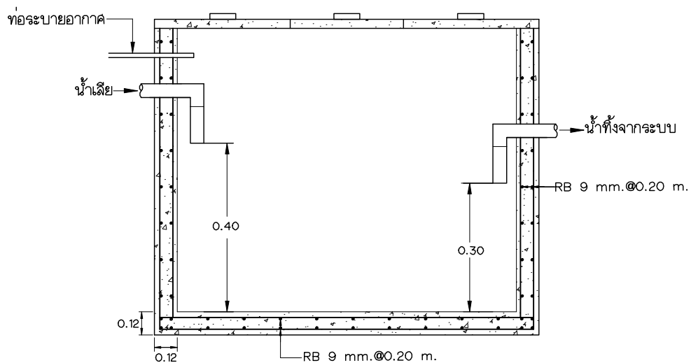
บ่อดักไขมันแบบสร้างในที่สำหรับอาคารขนาดใหญ่
